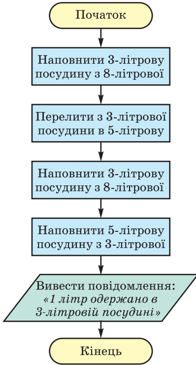
Рис. 2.3. Блок-схема алгоритму розв'язування задачі 1
