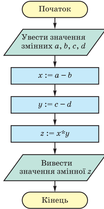
Рис. 2.4. Блок-схема алгоритму розв'язування задачі 2
