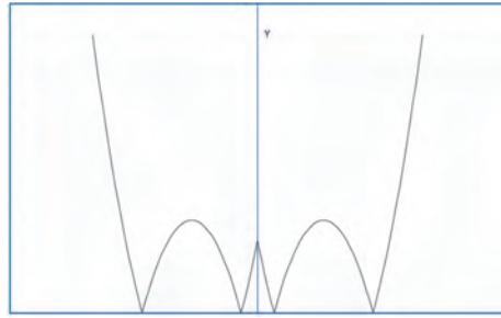
Рис. 1.9. Графік функції y = |x^2 - 8|x| + 7|
